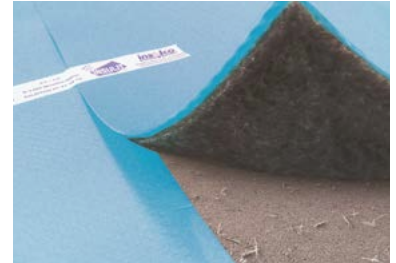
(1) Dérouler l'insulit 4+2 avec un recouvrement de 5 à 10 cm
